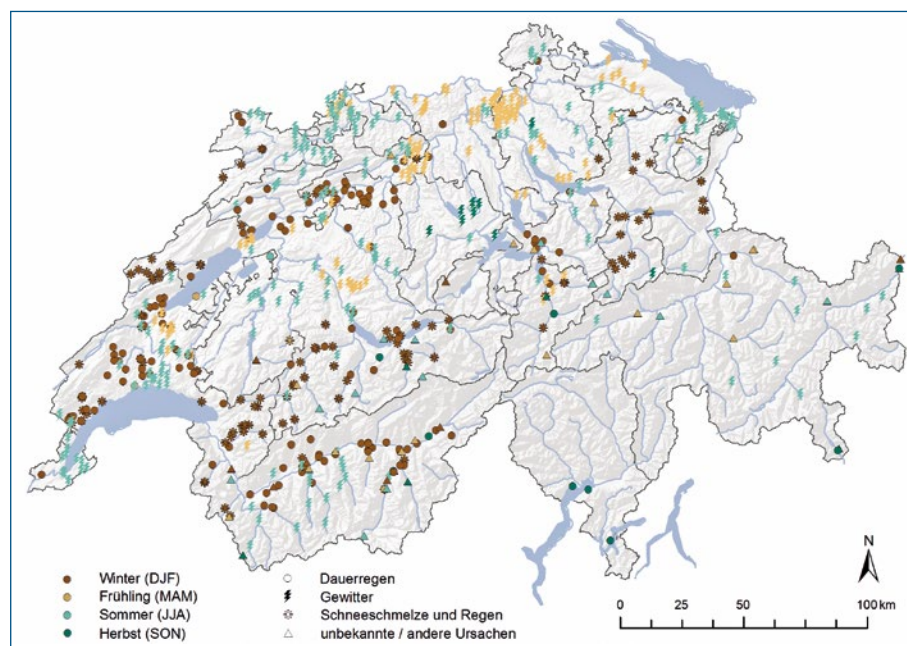
Bild 4. Oben: Ort, Ausmass und Prozessstyp der Schadensereignisse im Jahr 2018. Unten: Ort, Saison und meteorologische Ursache der Schadensereignisse im Jahr 2018 (Kartengrundlage: BFS GEOSTAT / Bundesamt für Landestopografie).
